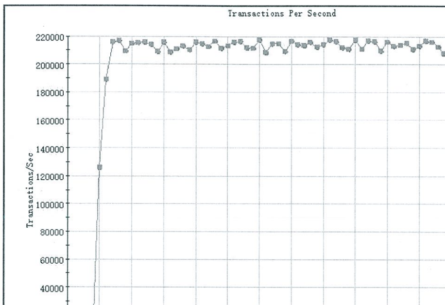
图 3 四层新建速率性能测试结果
