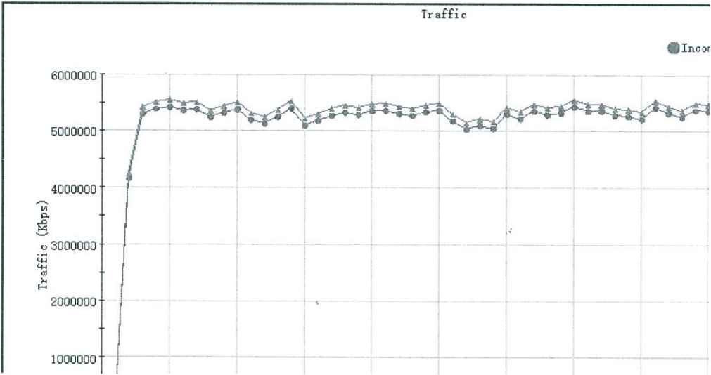
图 7 SSL 吞吐量性能测试结果
