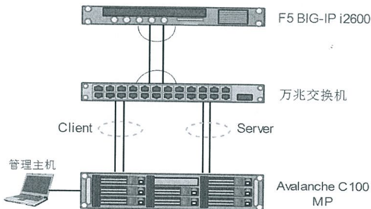
图 1 F5 BIG-IP i2600 应用交付设备性能测试环境示意图
