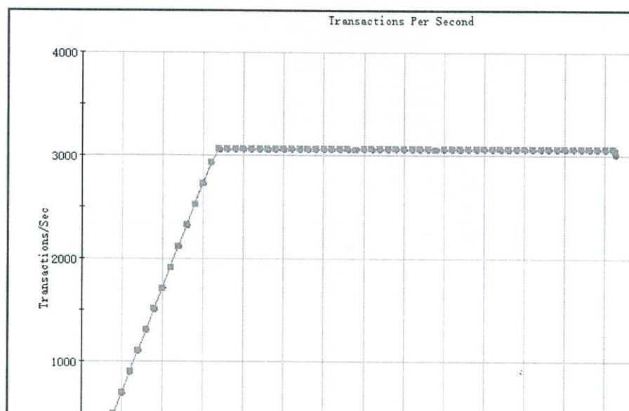
图 9 SSL 新建速率性能测试结果
