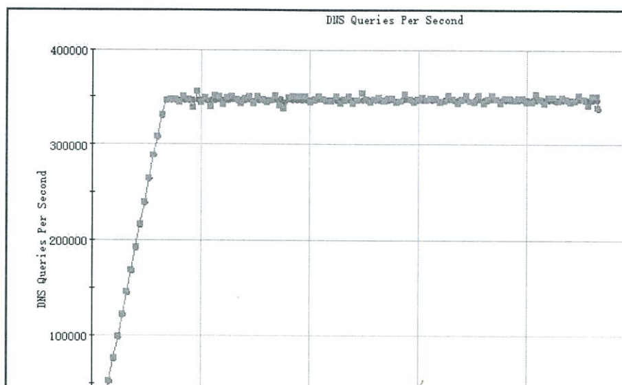
图 11 DNS 查询响应速率性能测试结果
