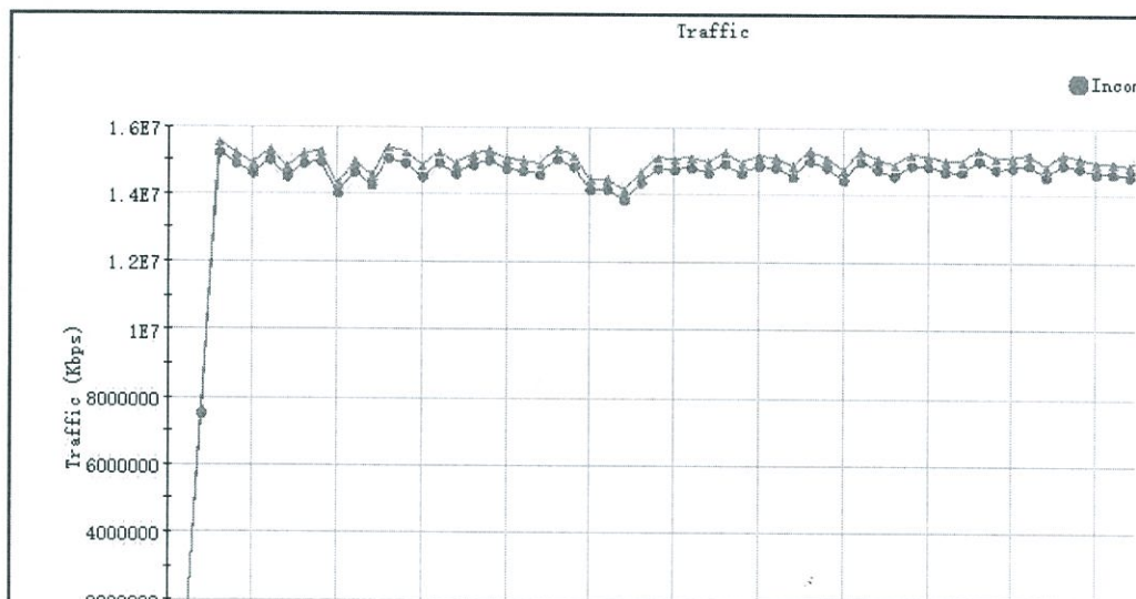
图 5 七层吞吐量性能测试结果
