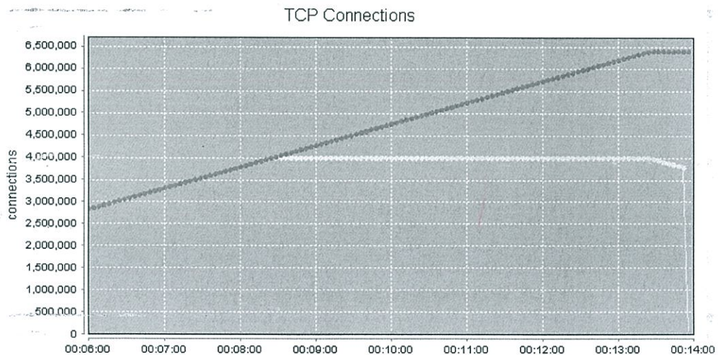
图 10 SSL 并发连接数性能测试结果
