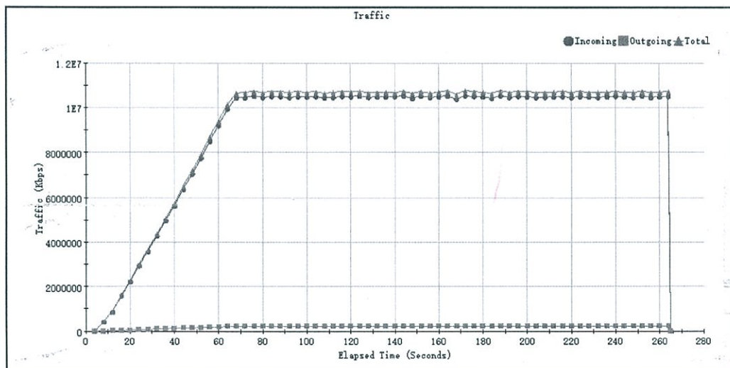
图 7 SSL 吞吐量性能测试结果
