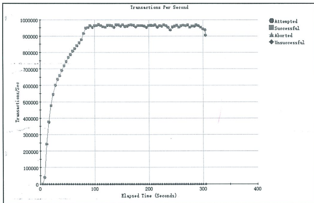
图 6 七层新建速率（每个连接中进行 20 次请求）性能测试结果
