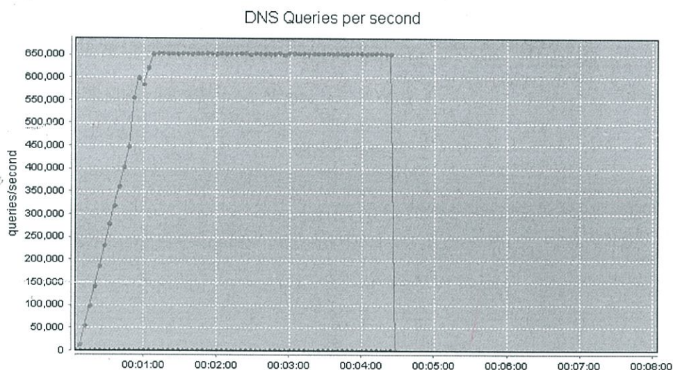
图 11 DNS 查询响应速率性能测试结果
