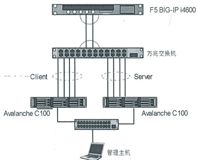
图 1 F5 BIG-IP i4600 应用交付设备性能测试环境示意图
