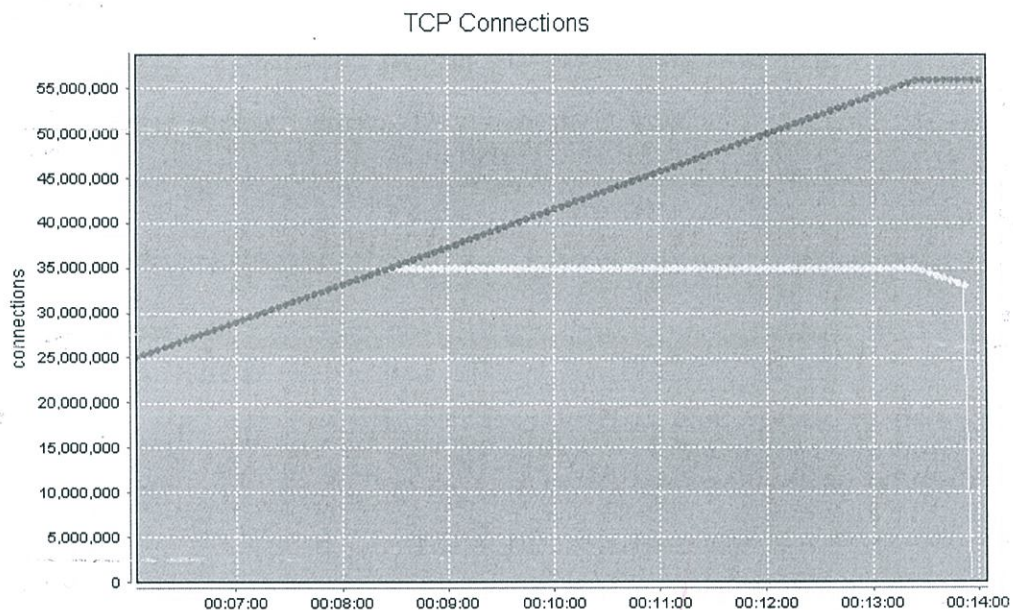
图 4 四层并发连接数性能
