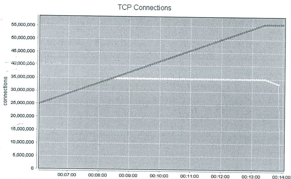
图 4 四层并发连接数性能
