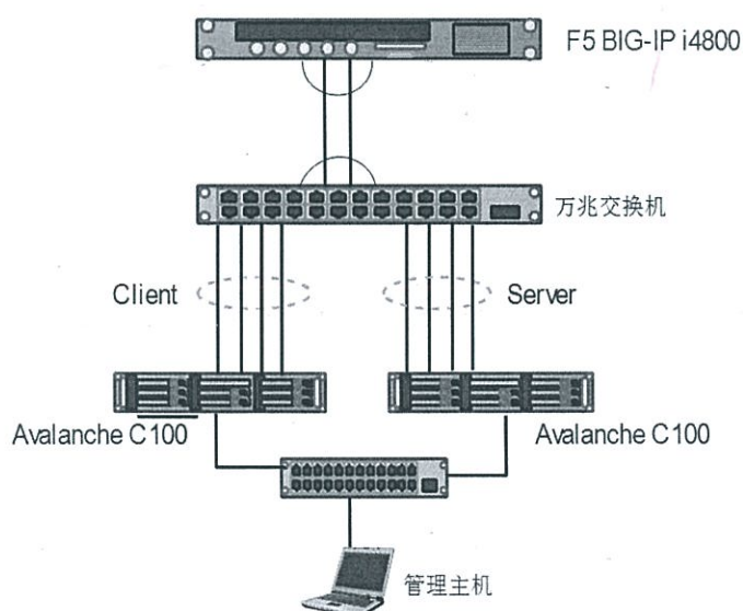
图 1 F5 BIG-IP i4800 应用交付设备性能测试环境示意图
