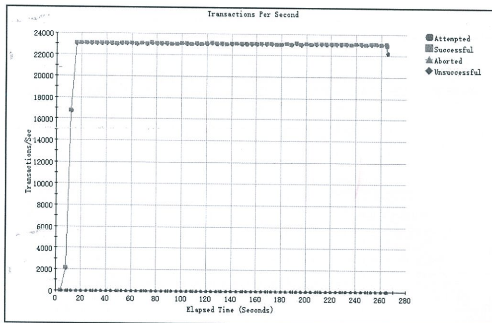
图 8 SSL 新建速率性能测试结果
