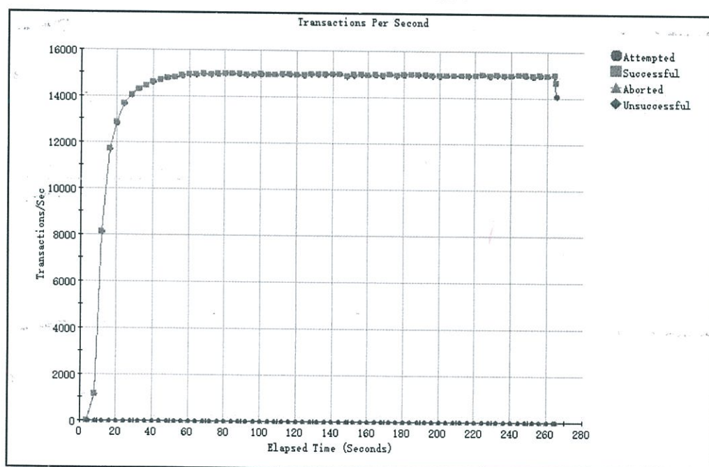
图 9 SSL 新建速率性能测试结果
