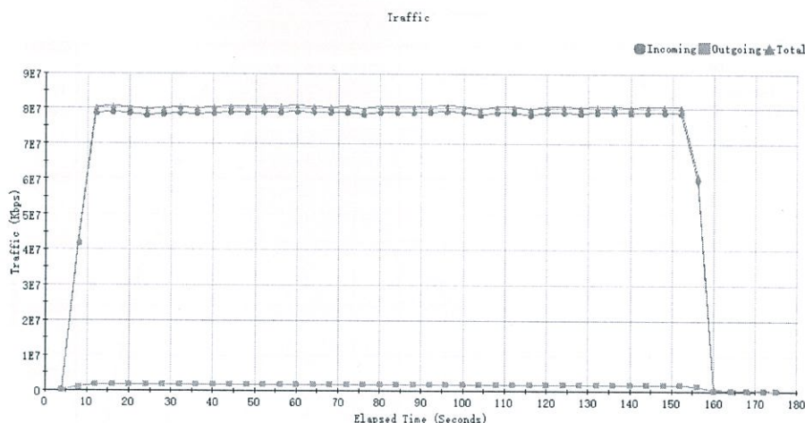
图 2 四层吞吐量性能测试结果
