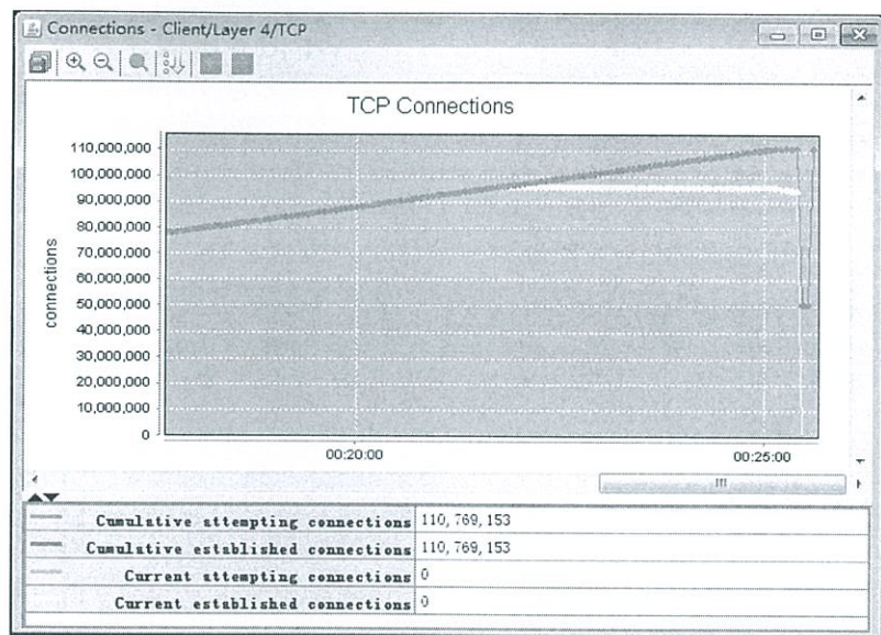
图 4 四层并发连接数性能
