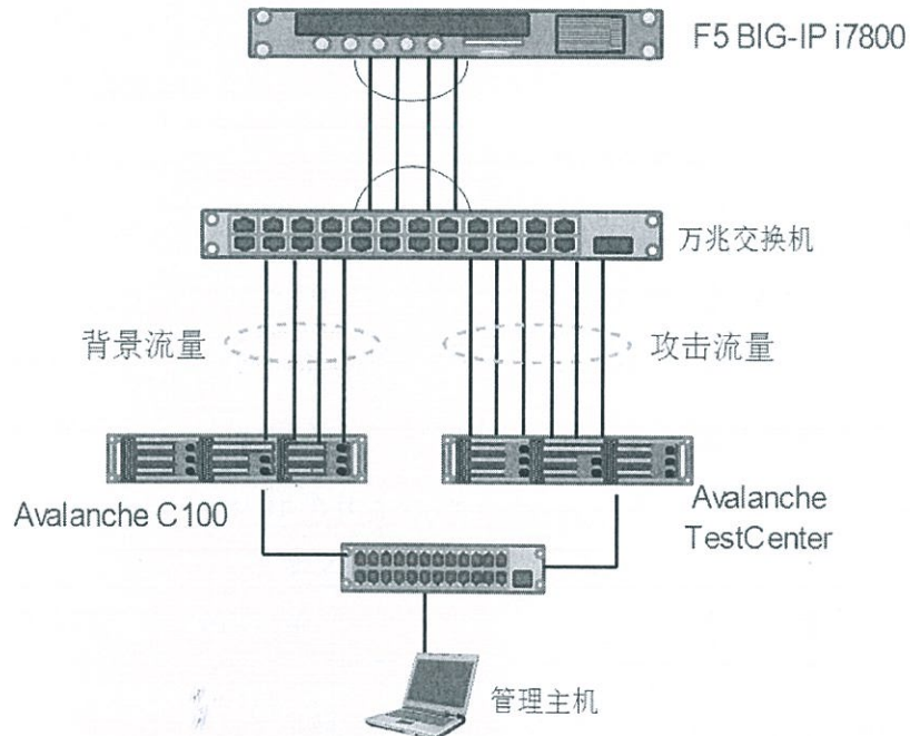
图 2 F5 BIG-IP i7800 应用交付设备 Synflood 攻击测试环境示意图
