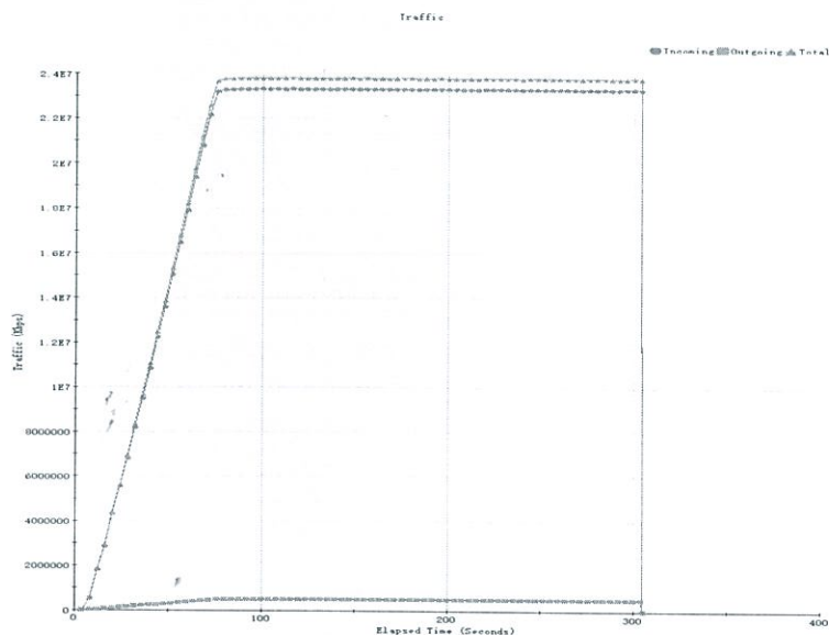
图 7 SSL 吞吐量性能测试结果
