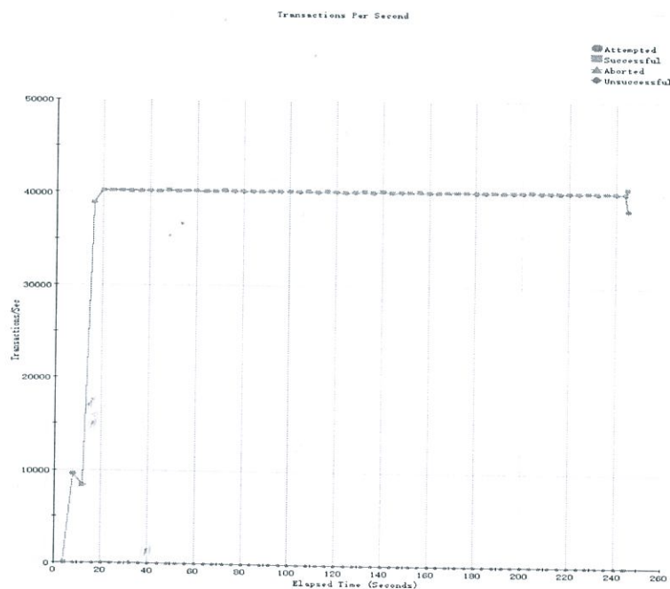
图 8 SSL 新建速率性能测试结果
