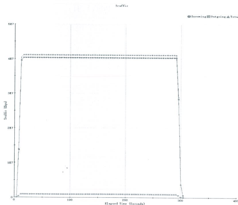
图 5 七层吞吐量性能测试结果
