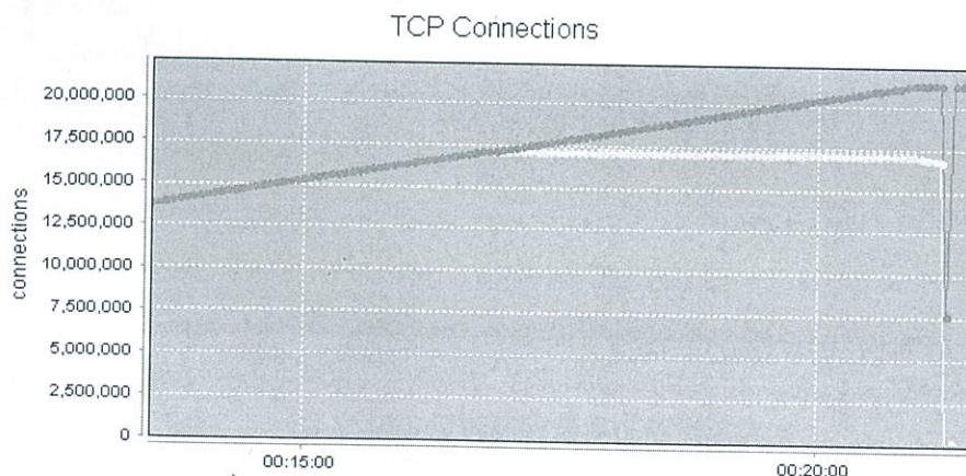
图 10 SSL 并发连接数性能测试结果
