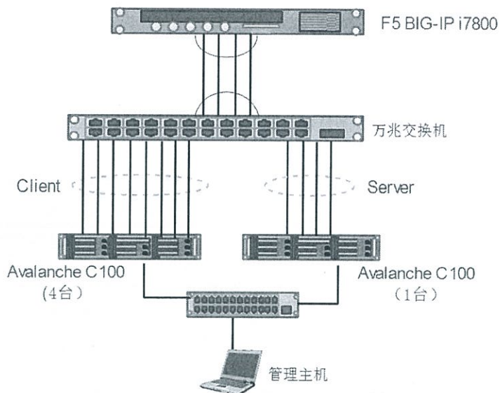
图 3 F5 BIG-IP i7800 应用交付设备 SSL 并发连接数测试环境示意图
