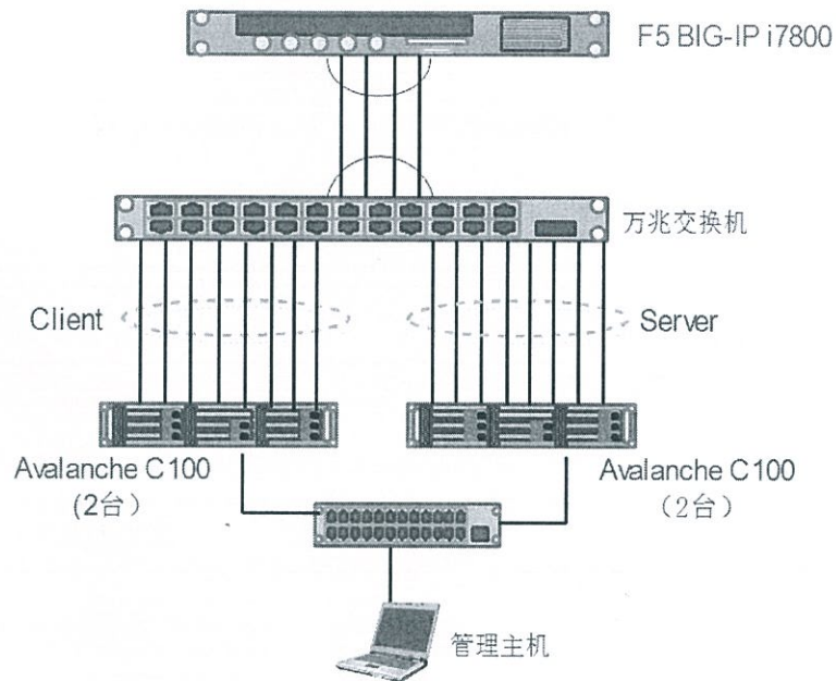
图 1 F5 BIG-IP i7800 应用交付设备性能测试环境示意图
