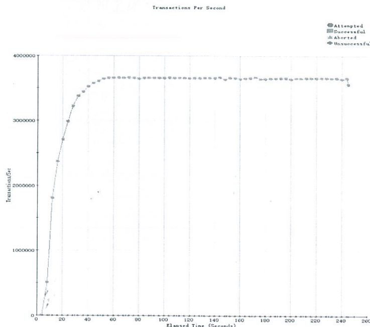
图 6 七层新建速率（每个连接中进行 100 次请求）性能测试结果
