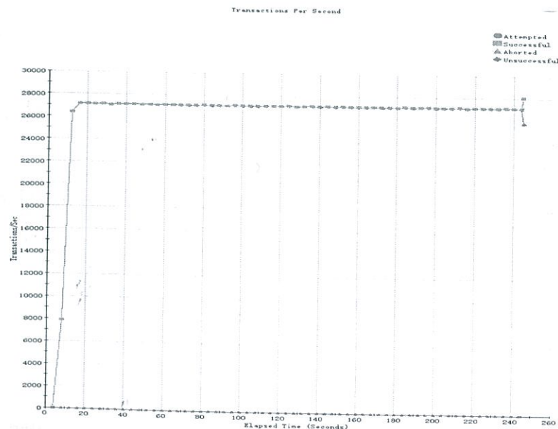
图 9 SSL 新建速率性能测试结果
