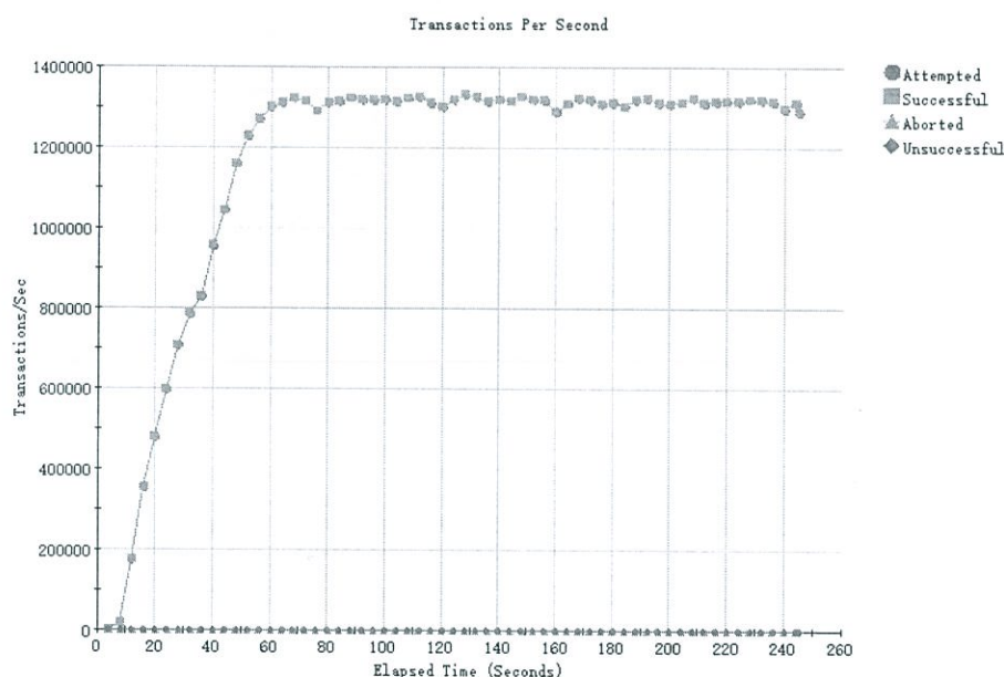
图 3 四层新建速率性能测试结果
